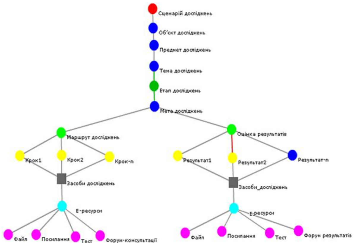
Рис. 1. Загальна граф-орієнтована структура онтологічної моделі е-сценарію супроводу процесу наукових досліджень учнями МАНУ
